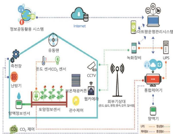
그림49 스마트팜 구성도
