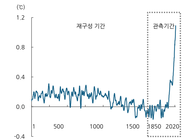
그림1 재구성기간(1~2000년) 관측기간 통합 기온 변화 추이
