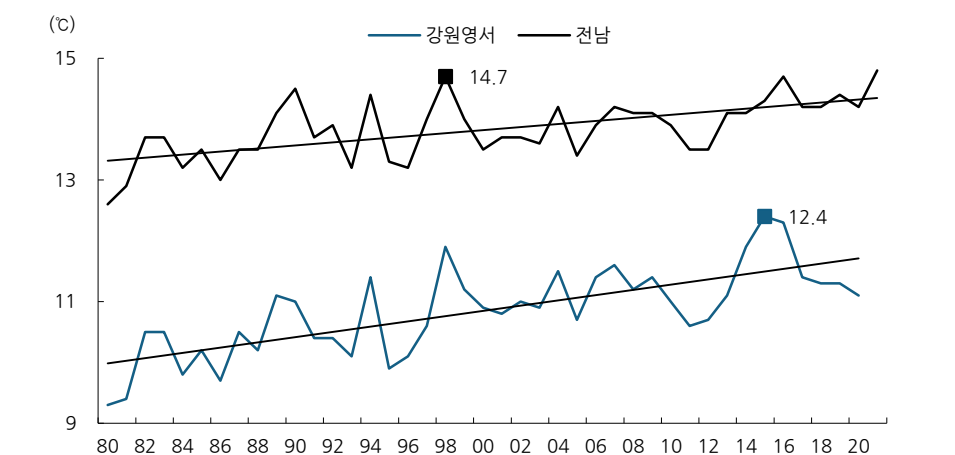
그림5 전남권, 강원영서권 연평균 기온 변화 추이 (1980년 ~ 2021년)
