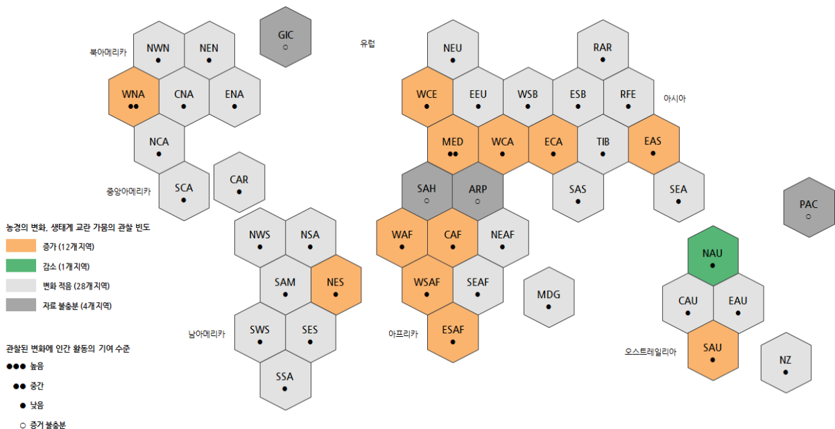
그림3 1950년 이후 농업과 생태계 교란 가뭄의 관찰된 변화
