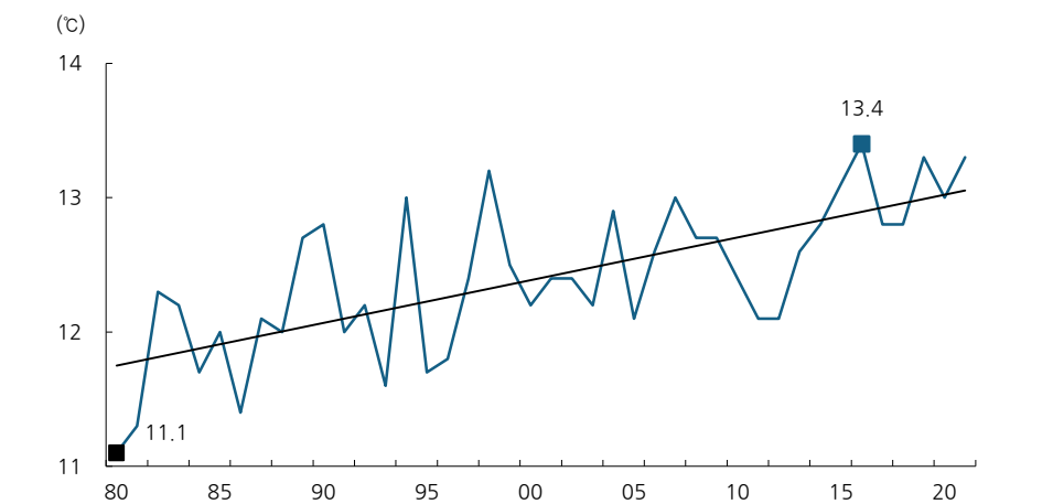
그림4 전국 연평균 기온 변화 추이 (1980년 ~ 2021년)
