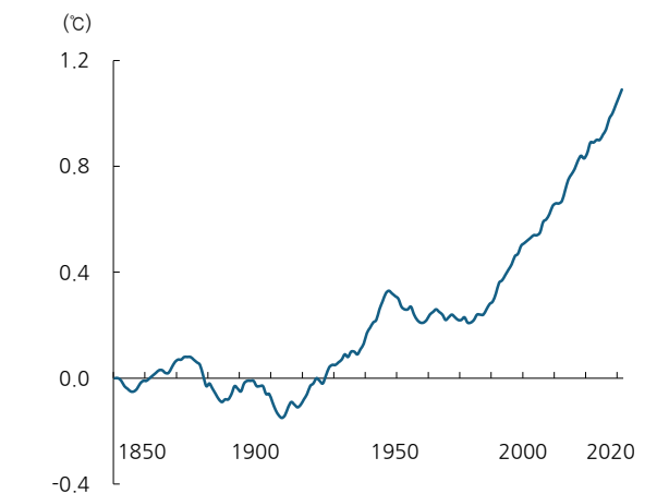
그림2 관측기간(1850년 이후) 기온 변화 추이
